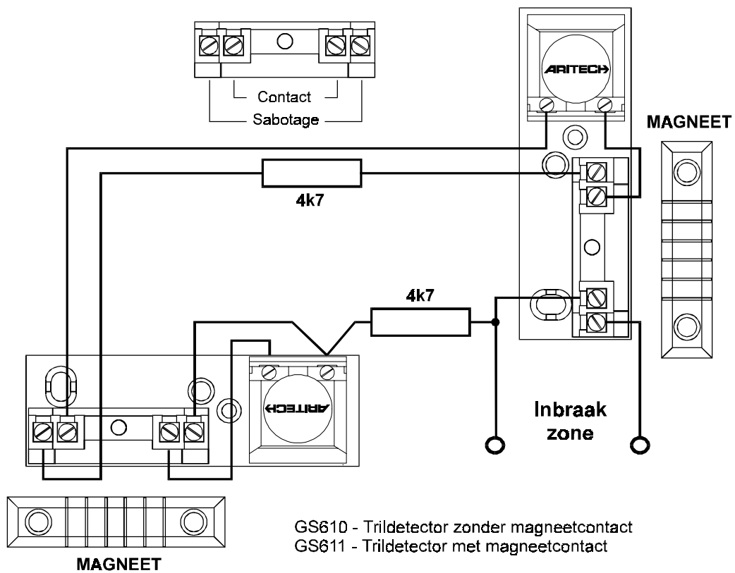
Figuur 26a. Aansluiting van de GS610/611 met gezamenlijke Alarm & Sabotage lus
