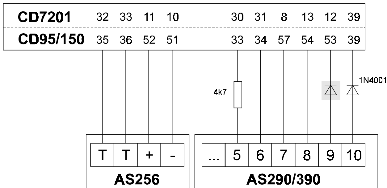
Figuur 22. Aansluiting van de AS256 binnensirene en de AS294/394 buitensirene
