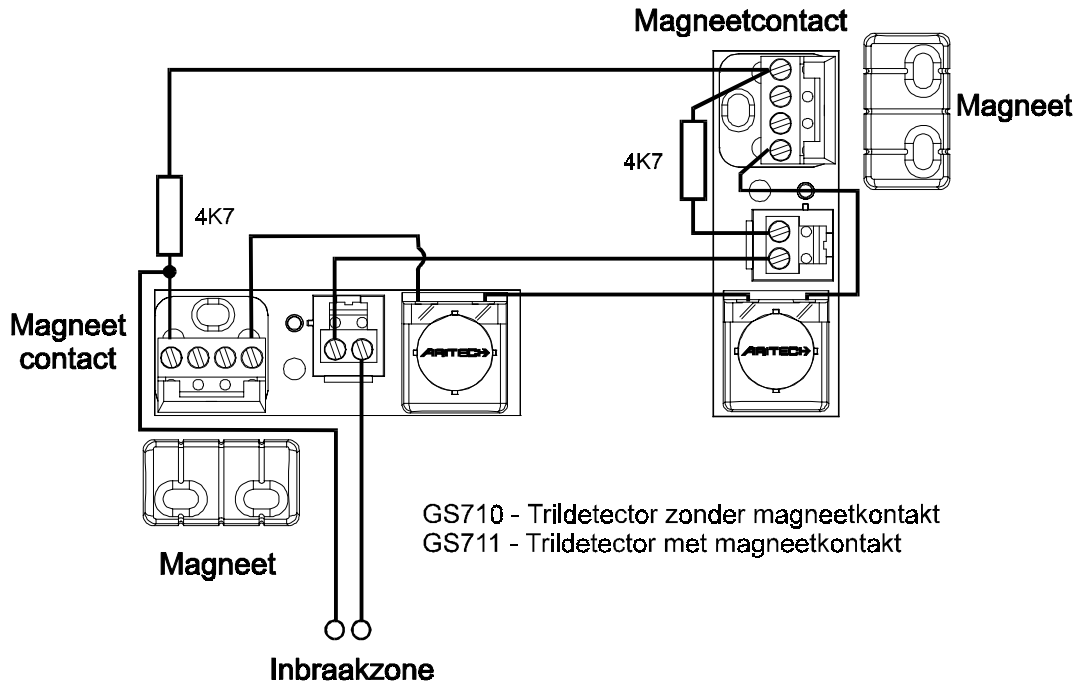
Figuur 26. Aansluiting van de GS710/711 met gezamenlijke Alarm & Sabotage lus
